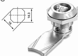
قفل زیمسنی مغزی مثلث سیلندر ۱۶ Quarter Turn Cam Lock 358
